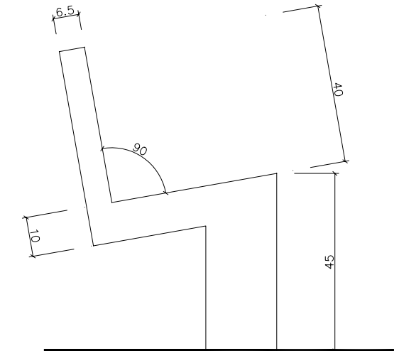
ALZADO LATERAL
